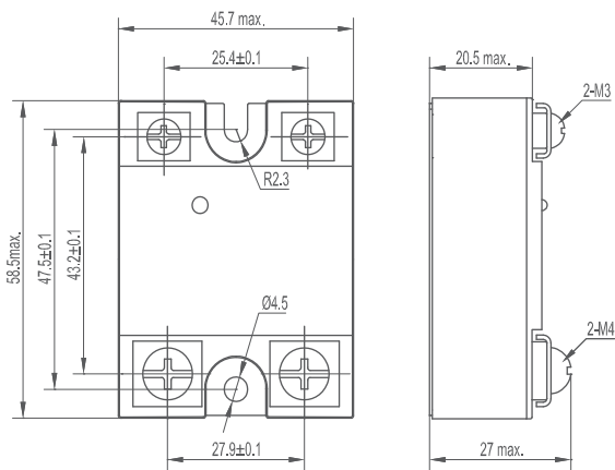
安装尺寸图
