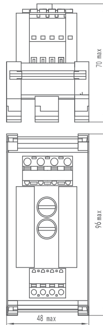
DRA-2系列尺寸图
