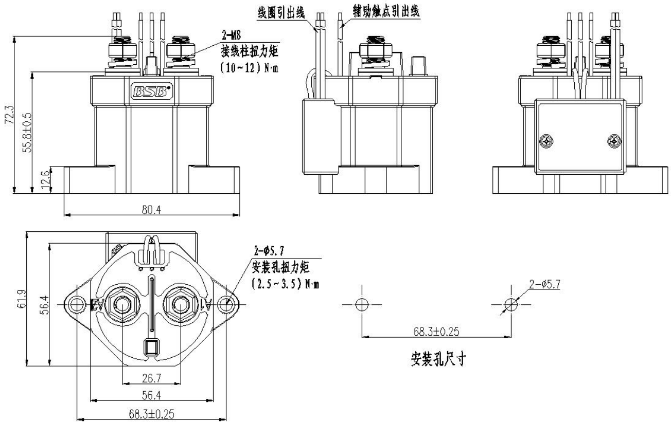
图 1 BSBC7-350B 产品外形及安装尺寸图
