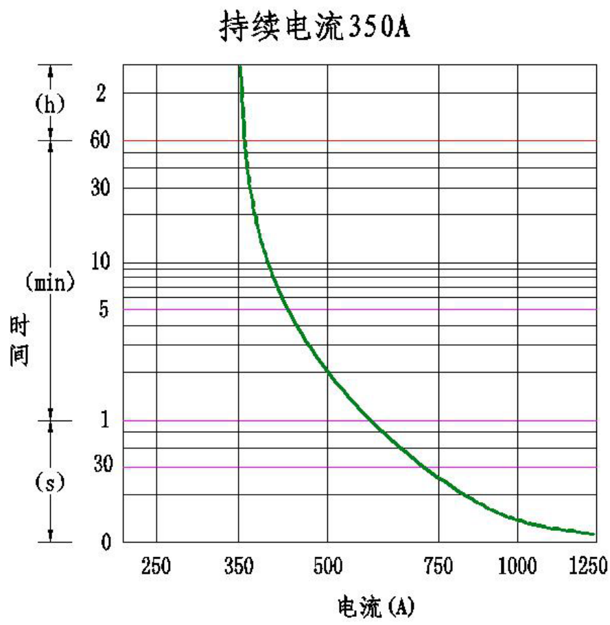
图1 短时过载能力曲线图
