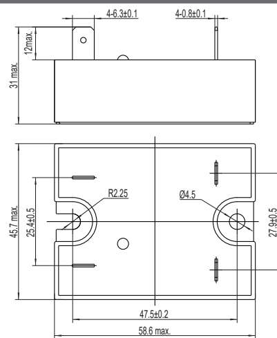
(016) 安装尺寸图
