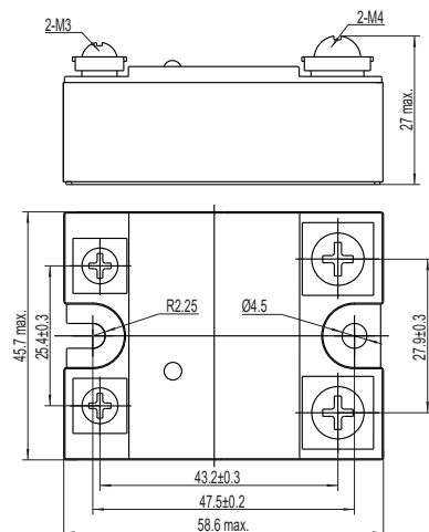
常规安装尺寸图
