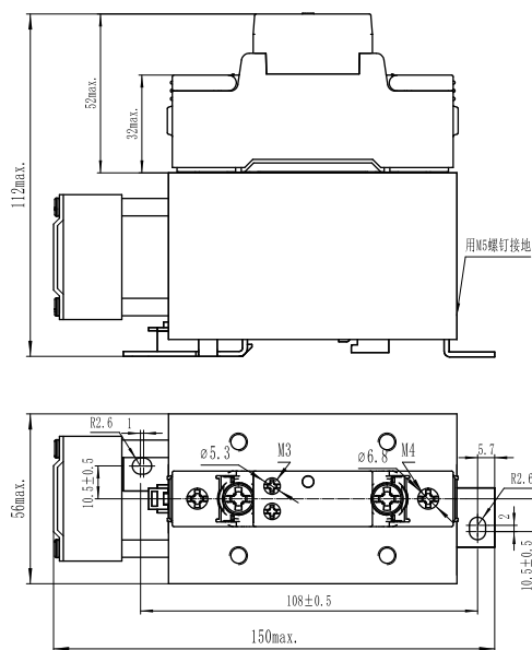
KSK...75...-IF24DC 系列
