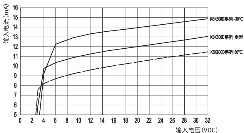
KSK600D... 系列
