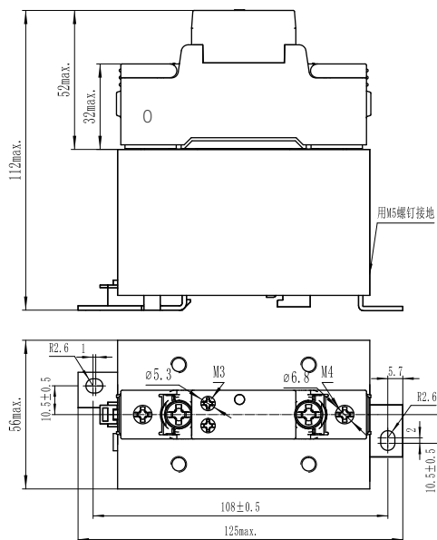
KSK...50...-I 系列
