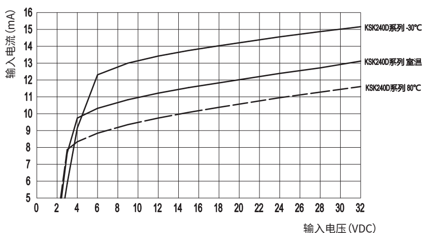
KSK240D... 系列
