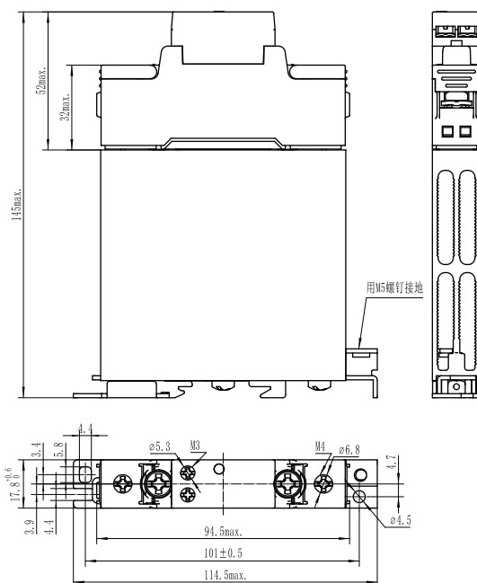
KSK...25/50...-L 系列
