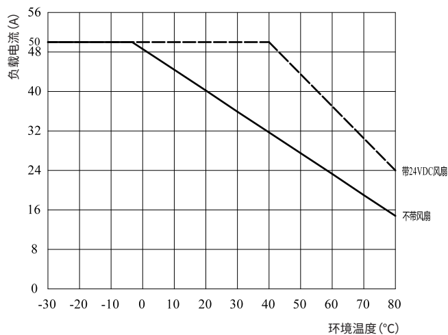
KSK...50...-I 系列
