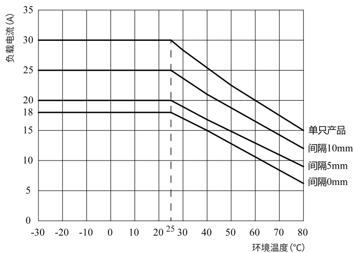
KSK...25...-K 系列
