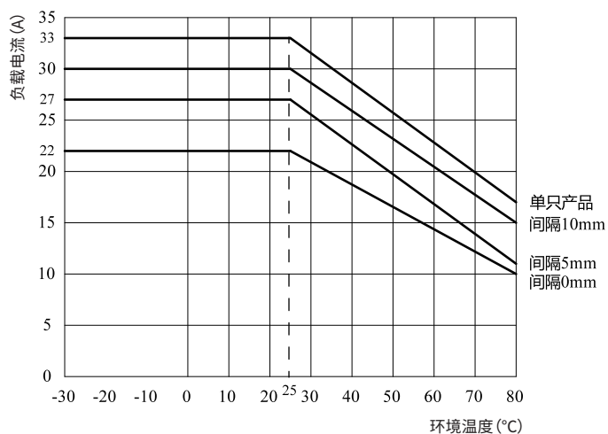
KSK...25...-L 系列
