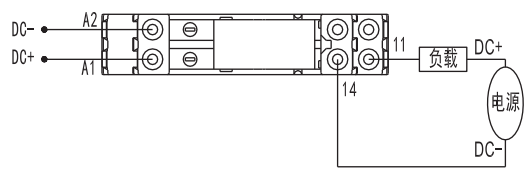
带底座产品
