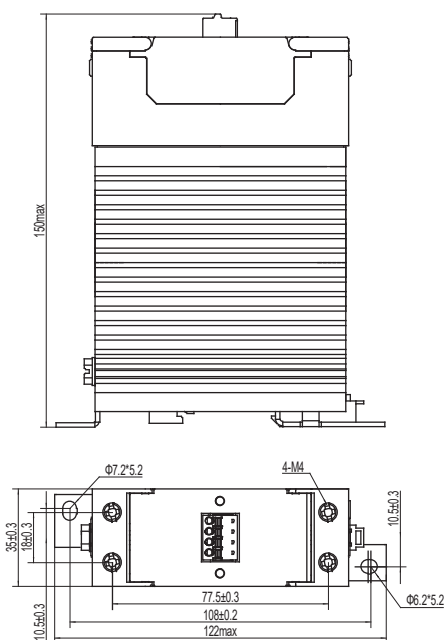
带KHS-H90散热器
