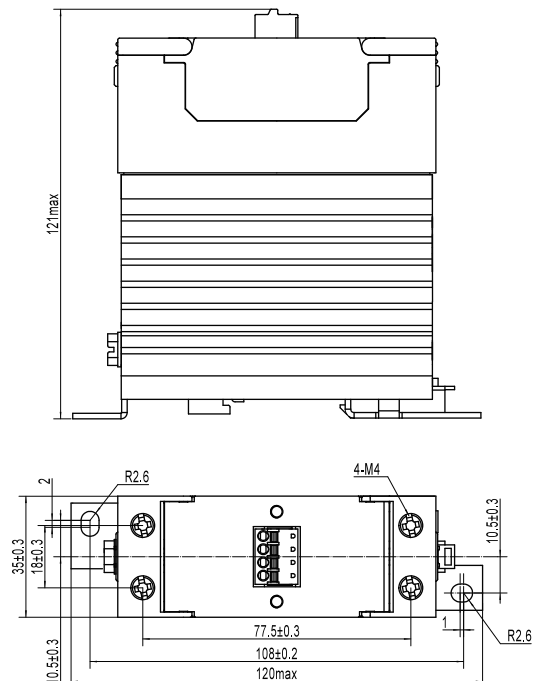
带KHS-P90散热器
