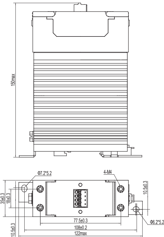
带KHS-H90散热器
