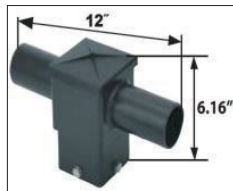
PKL-F2
