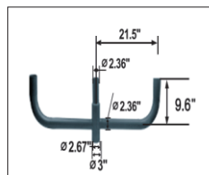
PKL-RL03
