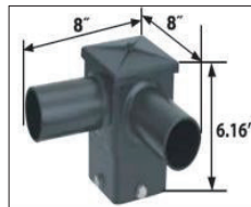
PKL-FC2
