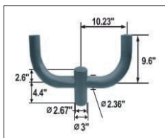
PKL-RL02
