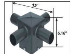
PKL-F4
