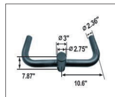
PKL-RU02
